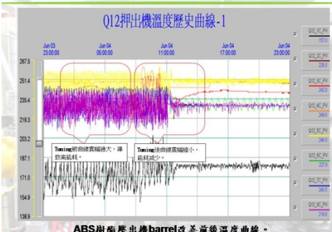
ABS樹脂壓出機barrel溫度控制最佳化
