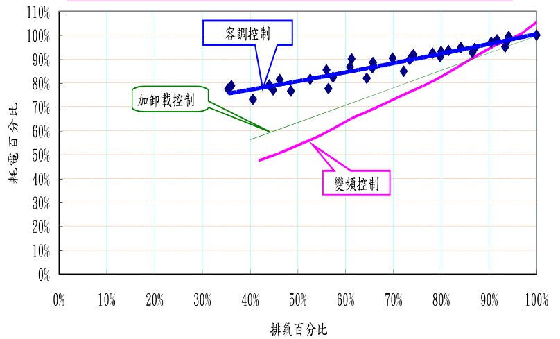
容調、加卸載與變頻控制之空壓機 在部分負載下的耗電比較圖
